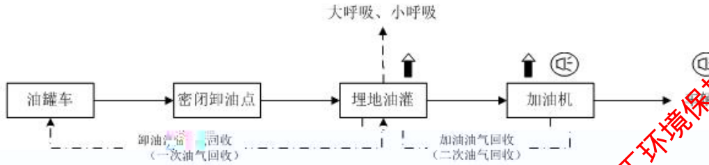
加油工艺流程及产污节点图
